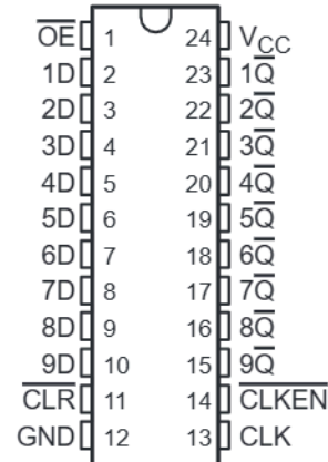
EN PACKAGE (TOP VIEW)
