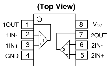
SO-8/TSSOP-8/MSOP-8
