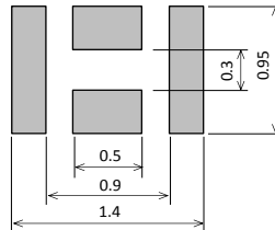
NFMJMPC
