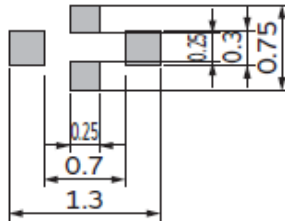
NFM18CC/18PC
