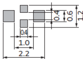
NFM21CC/21PC
