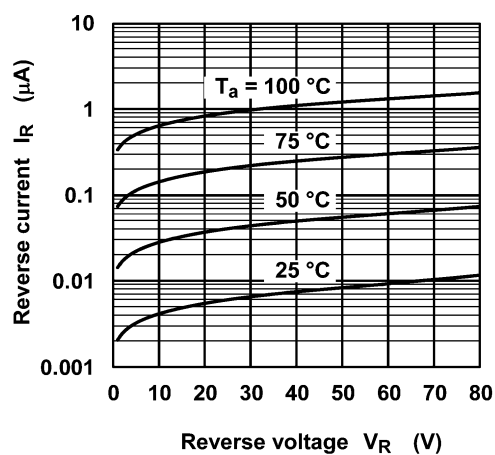
Fig. 7.2 I_R - V_R
