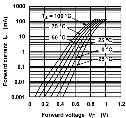
Fig. 7.1 I_F - V_F
